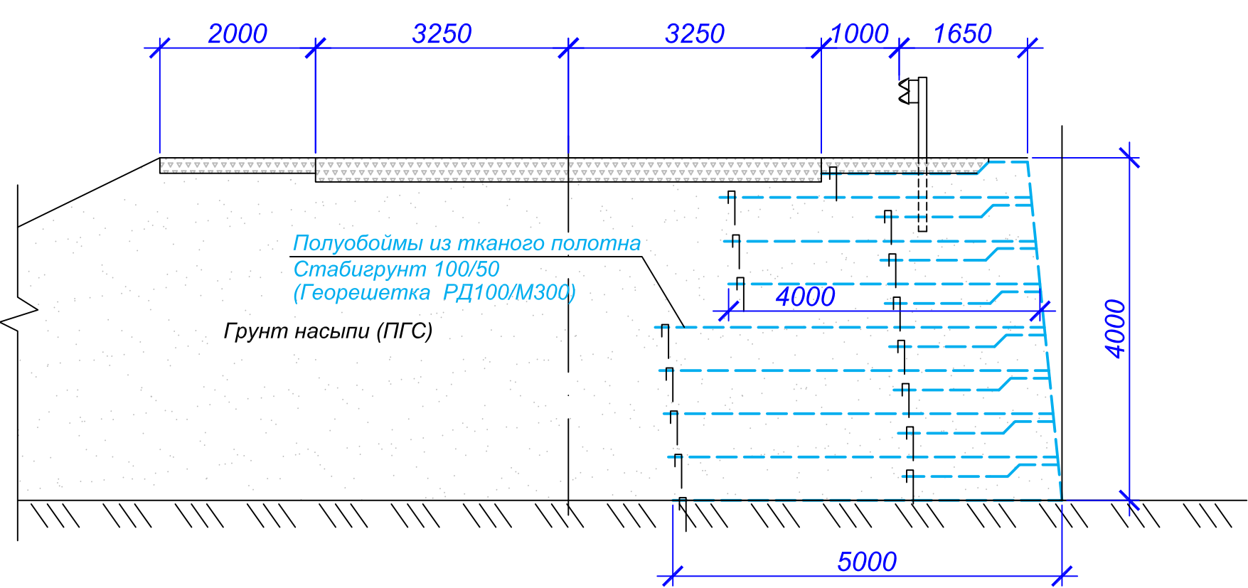
Варианты 3. По методу обертывания без облицовки
