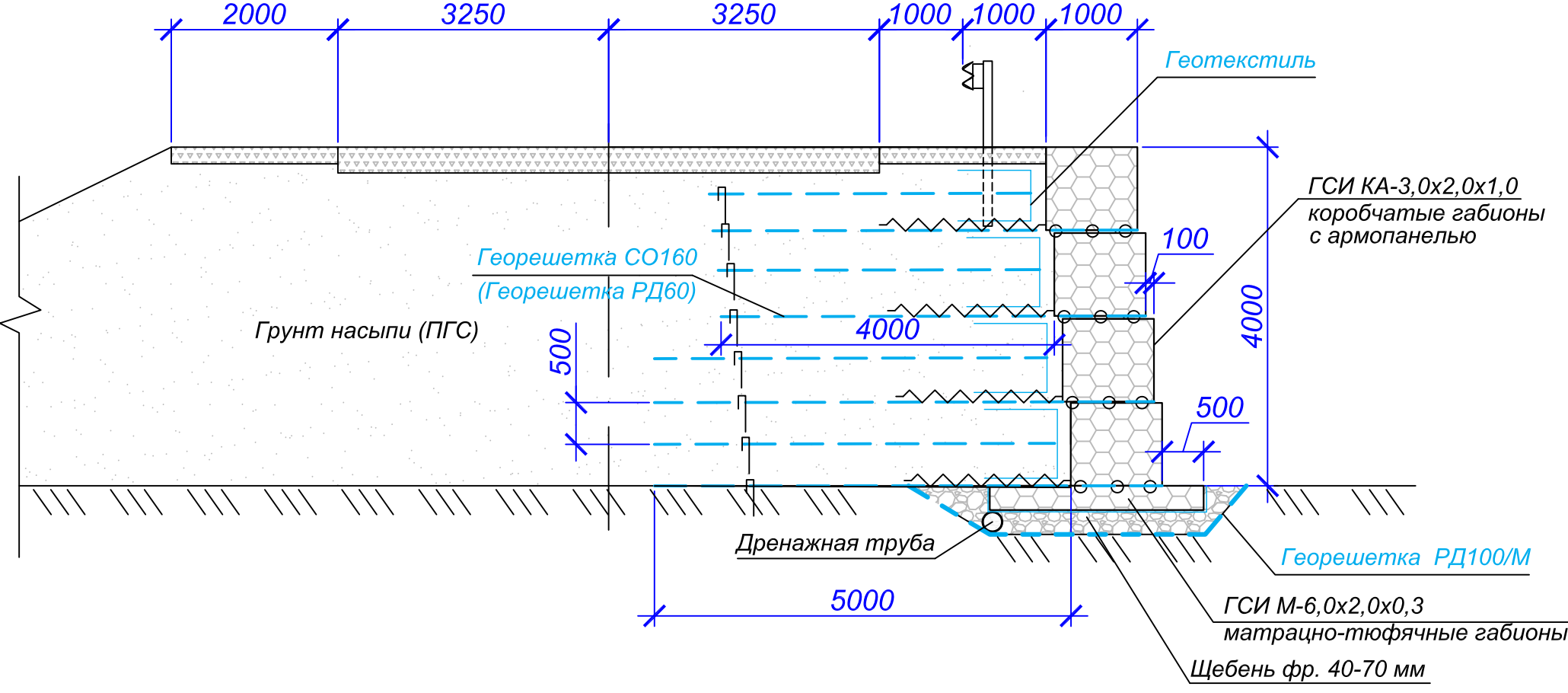
Варианты 2. С облицовкой из габионов
