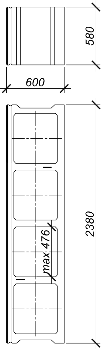
Бетонный пустотный блок типа ФБП по ГОСТ 13579-78
