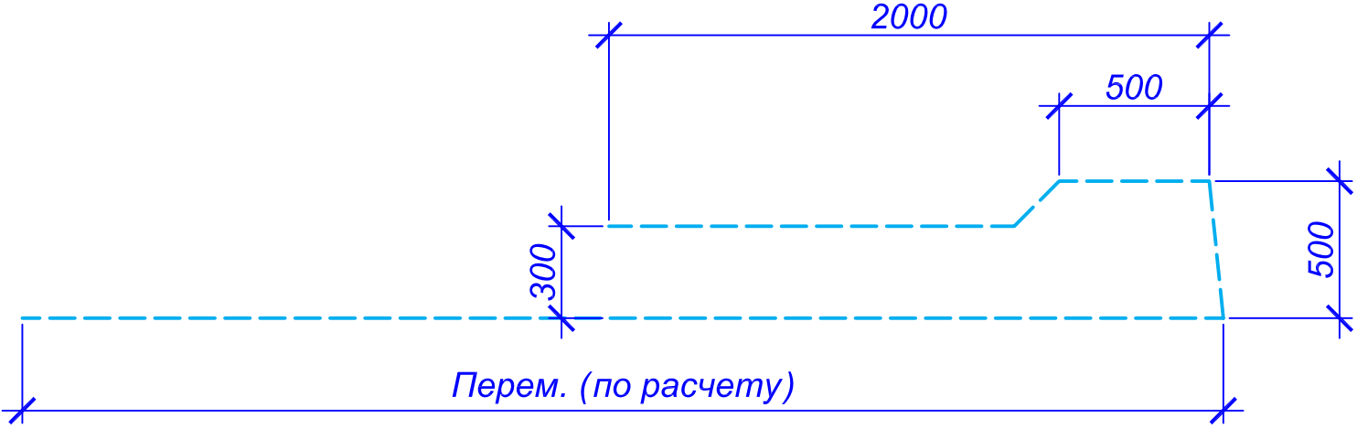
Полуобойма из тканого полотна (плоской георешетки с подложкой)
