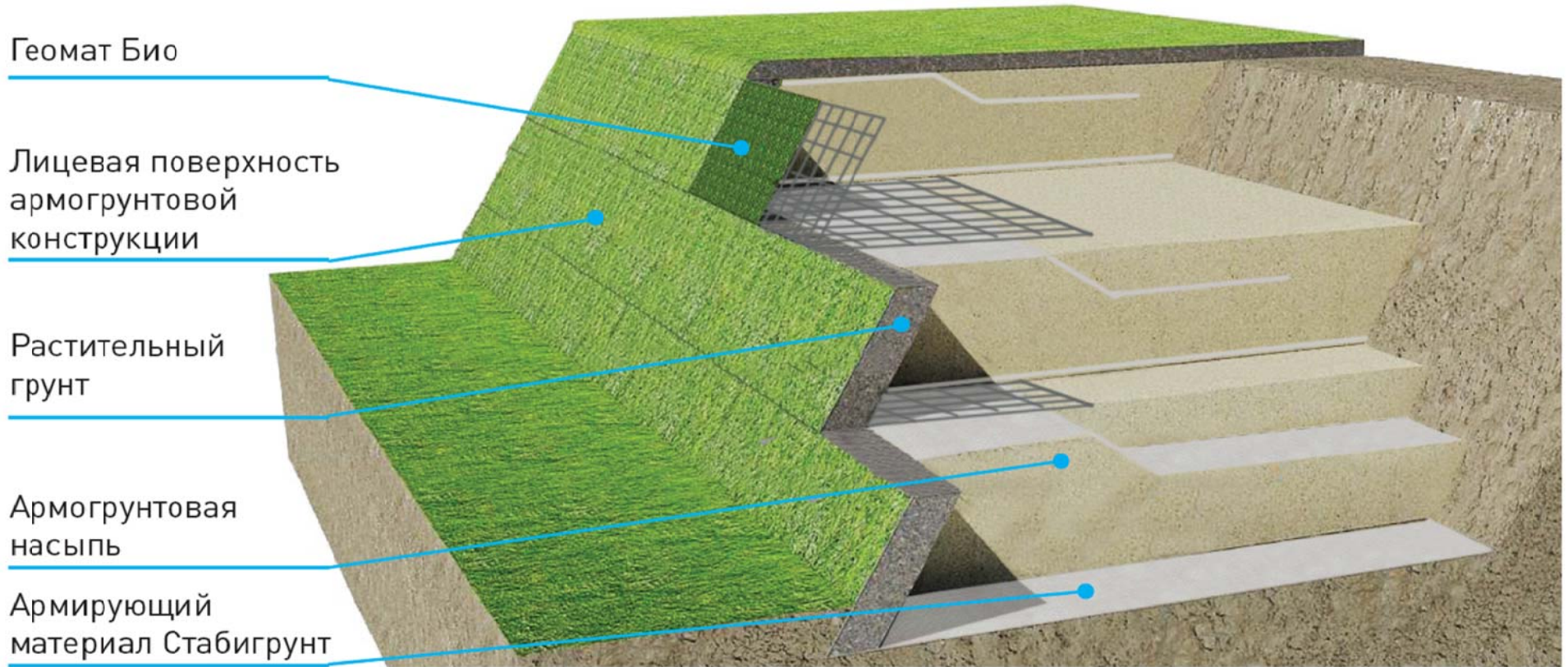
Подпорная стена по методу обертывани
