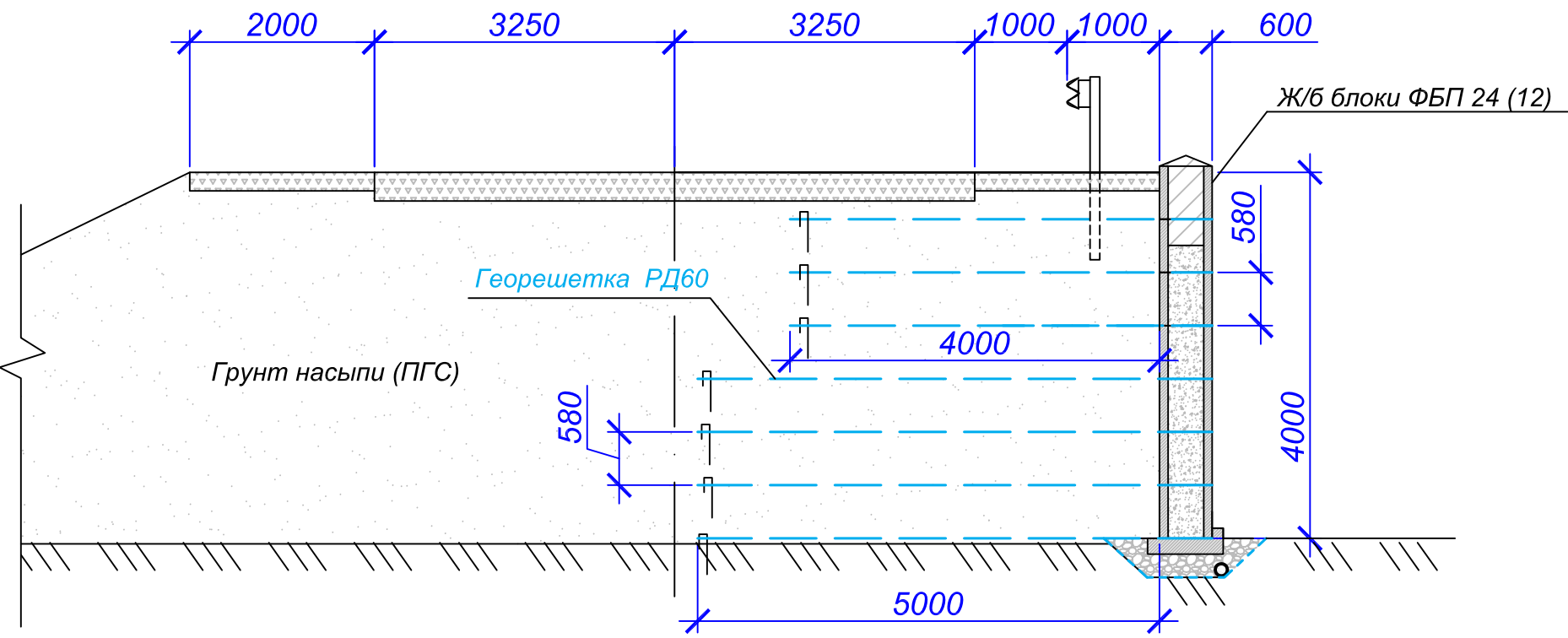
Варианты 1. С облицовкой из ж/б блоков
