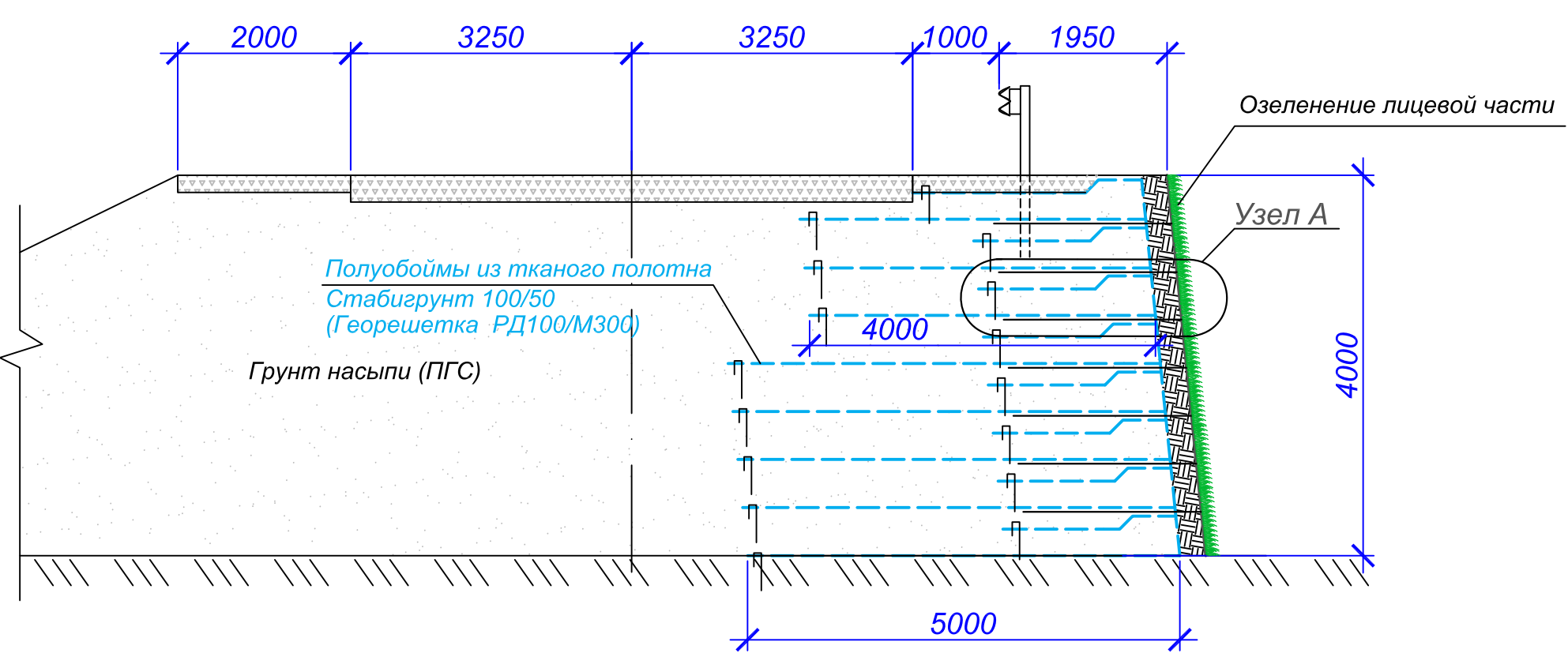
Варианты 4. По методу обертывания с озеленением лицевой части
