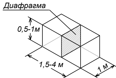
Конструкция габиона по ГОСТ Р 52132-2003
